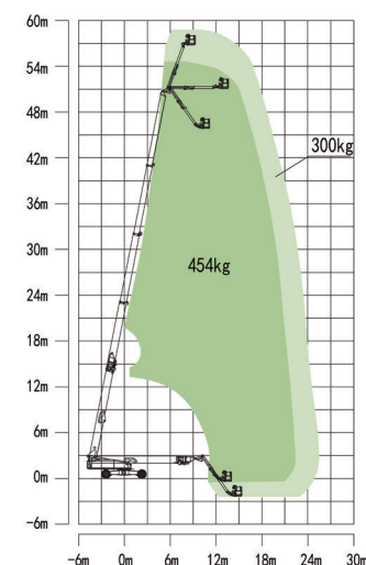
Courbes de travail ZT58J
