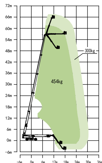
Courbes de travail ZT68J
